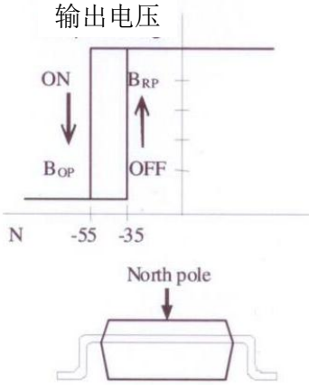
磁通密度 (高斯)
