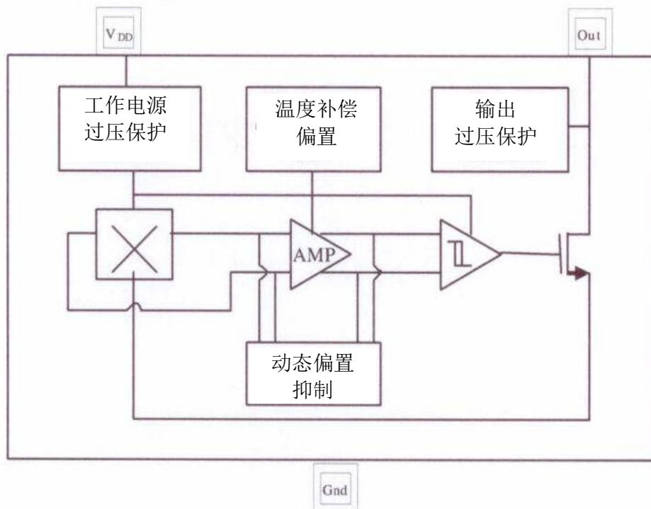
Fig. 1 功能框图
