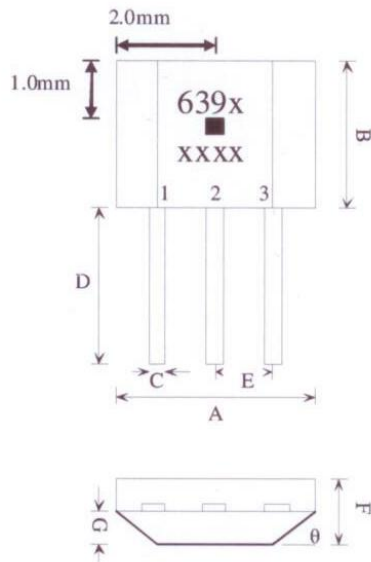
仰视图
