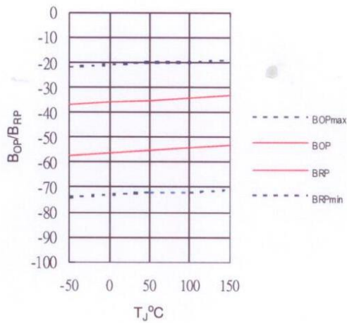
B_{OP} 和 B_{RP} 与温度关系
