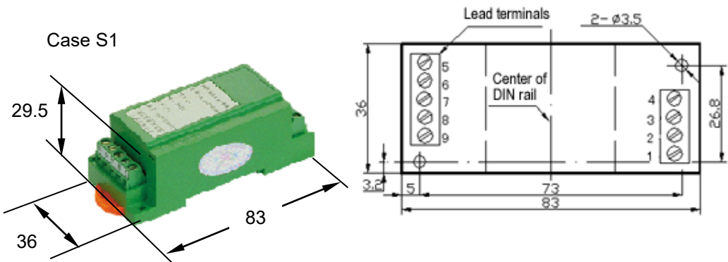
传感器尺寸: 29.5mm x 83mm x 36mm
