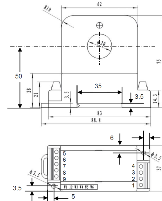
Abb. 2 Gehäuseabmessungen.
