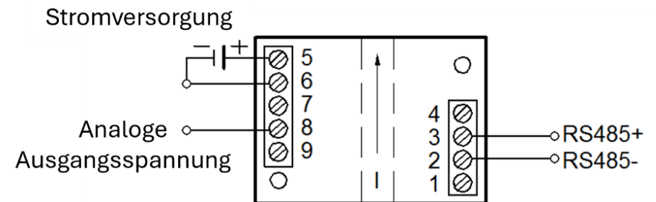
Abb. 3 Pinbelegung.
