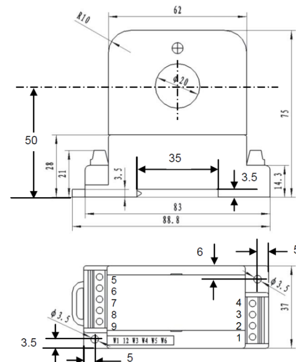
Abb. 3 Gehäuseabmessungen.
