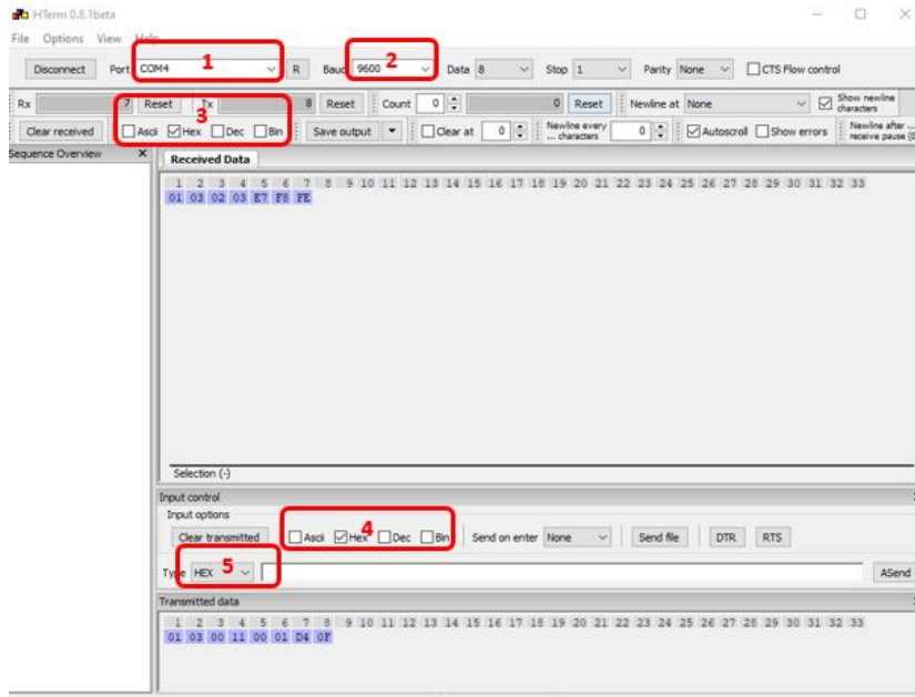
Abb. 6 HTerm-Parametereinstellungen.
