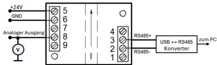
Abb. 5 Anschlussdiagramm des Sensors an das Mastergerät mit RS-485-Schnittstelle.
