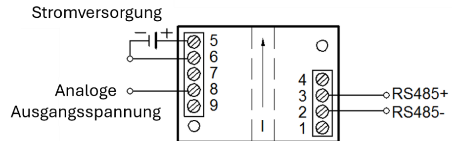
Abb. 3 Pinbelegung.
