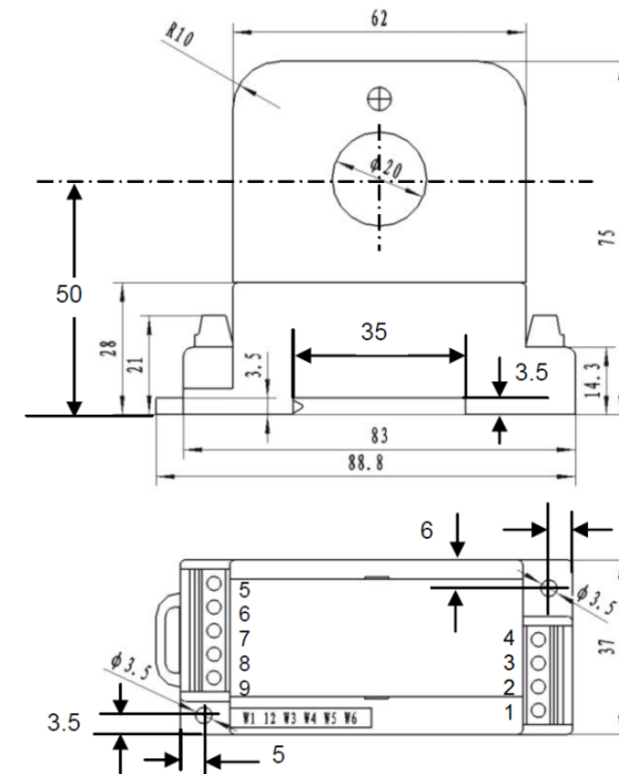
Abb. 2 Gehäuseabmessungen.
