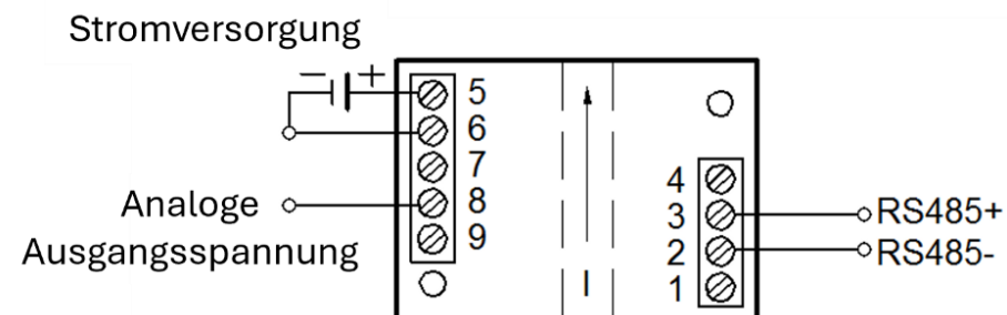
Abb. 3 Pinbelegung.
