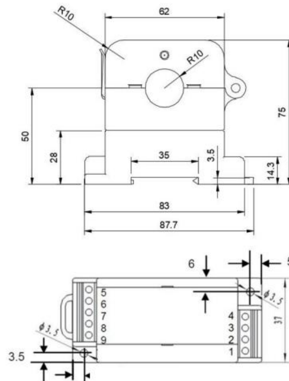
Abb. 2 Gehäuseabmessungen.
