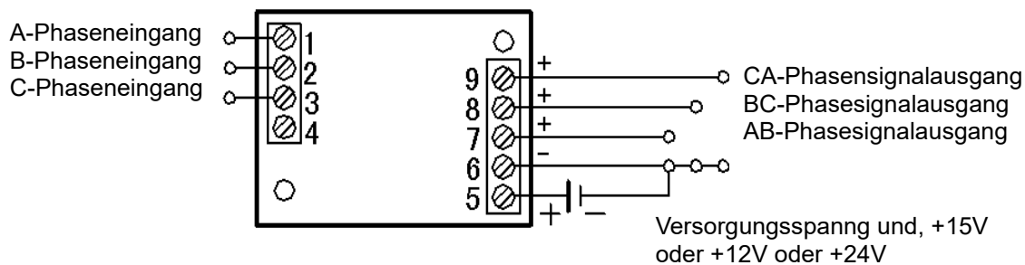
Dreiphasige 3-Draht AC Spannungssensor
